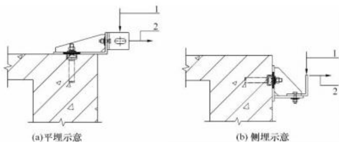
图 C.0.2 幕墙预埋系统现场拉拔检验示意
